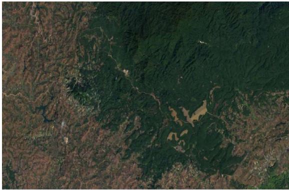
Hình 3.1. Tổ hợp màu 4,3,2 cảnh ảnh LC81240522014030LGN00
