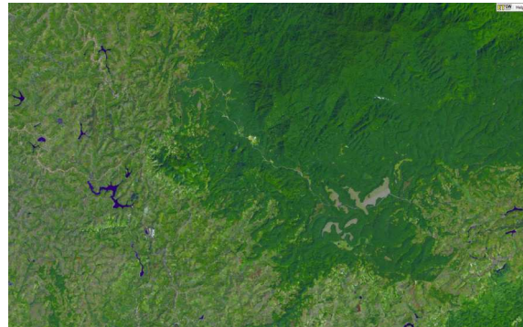
Hình 3.2. Tổ hợp màu 7,6,4 cảnh ảnh LC81240522014030LGN00
