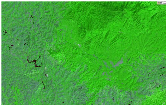
Hình 3.1. Tổ hợp màu 3,5,4 cảnh ảnh LC81240522014030LGN00
